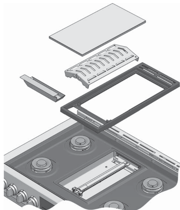
VUE ÉCLATÉE DU GRIL-BRÛLEUR
